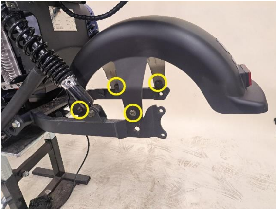
Irrota lokasuojan kiinnityspultit (kuusiokoloavain 5 mm).
