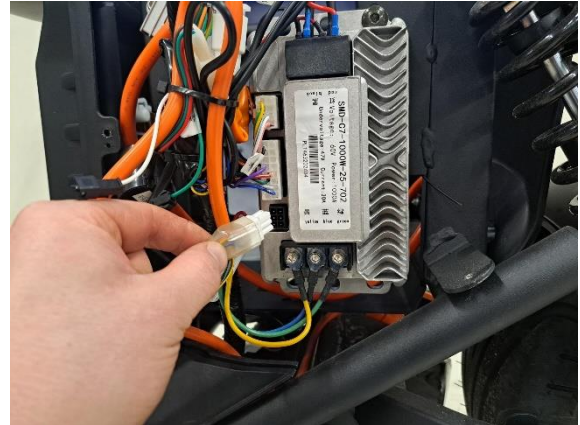
Irrota ohjainlaitteelta moottorin hall- antureiden liitin.
